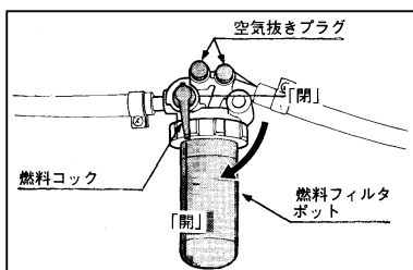
【燃料フィルター詳細図】
