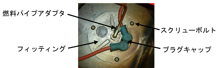
【ボイラーメンテパネル内部】
