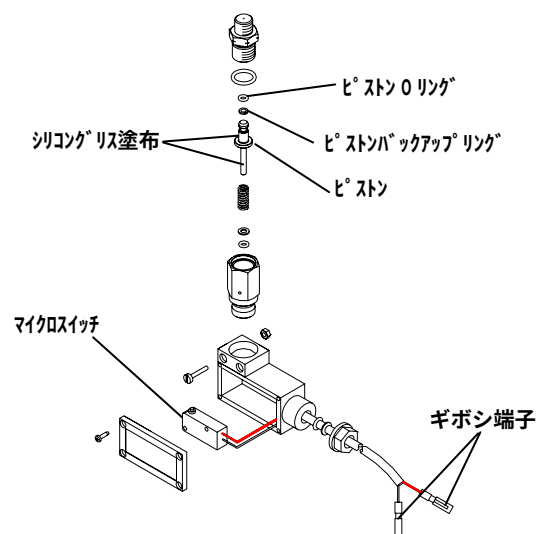
圧力スイッチ
