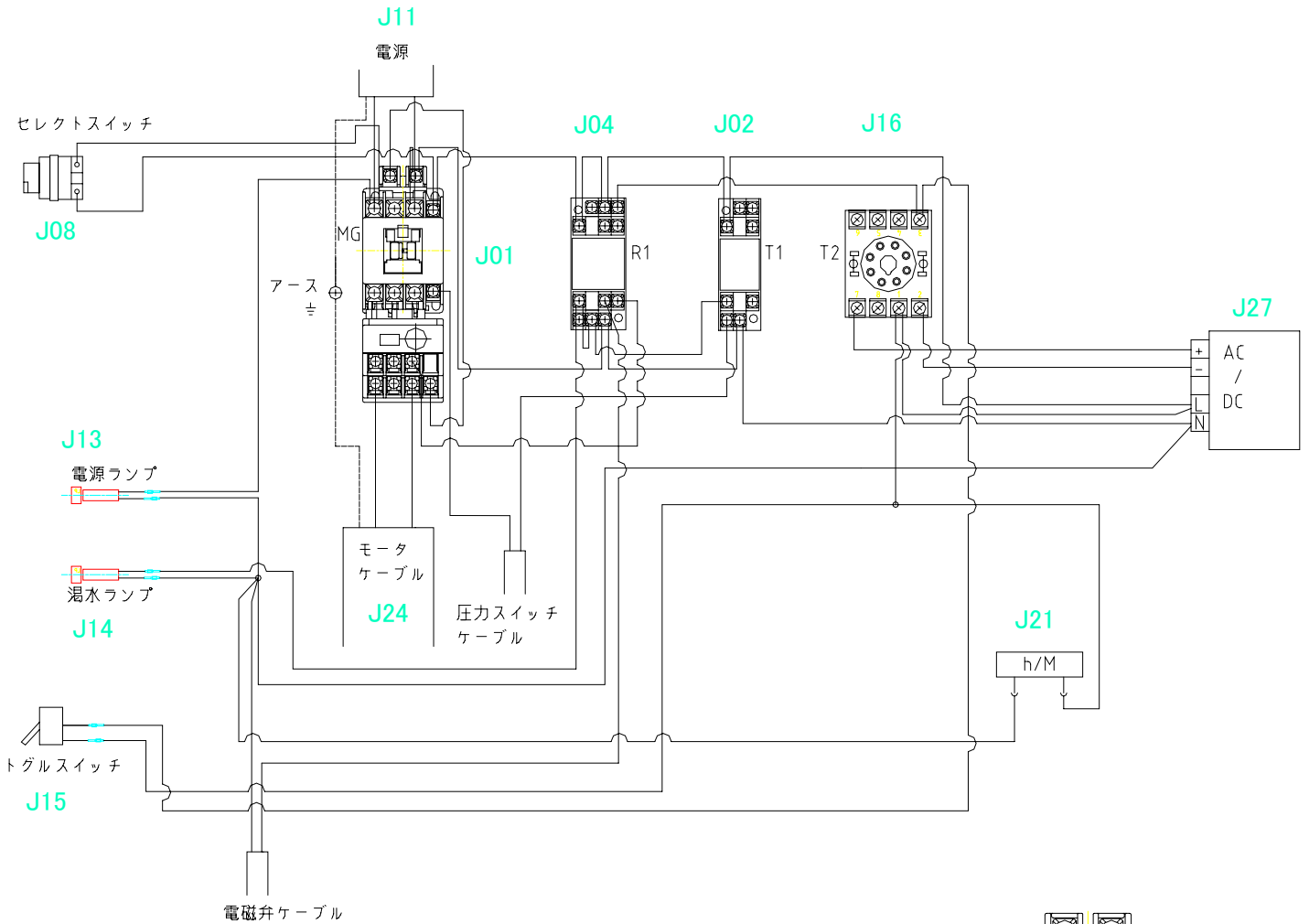
電磁開閉器
